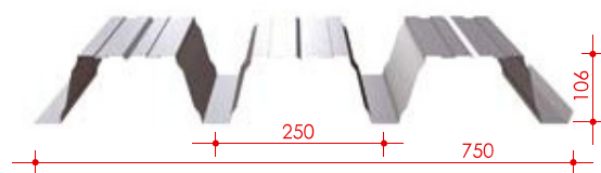
BTR 106 konstruksjonsprofil
