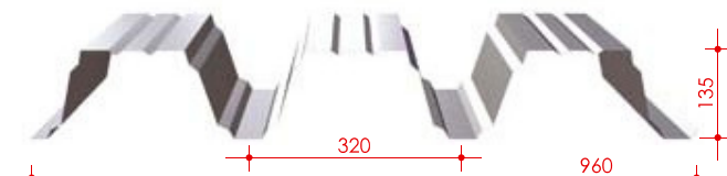
BTR 135 konstruksjonsprofil
