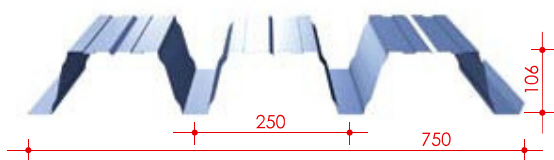
BTR 106 konstruksjon profil
